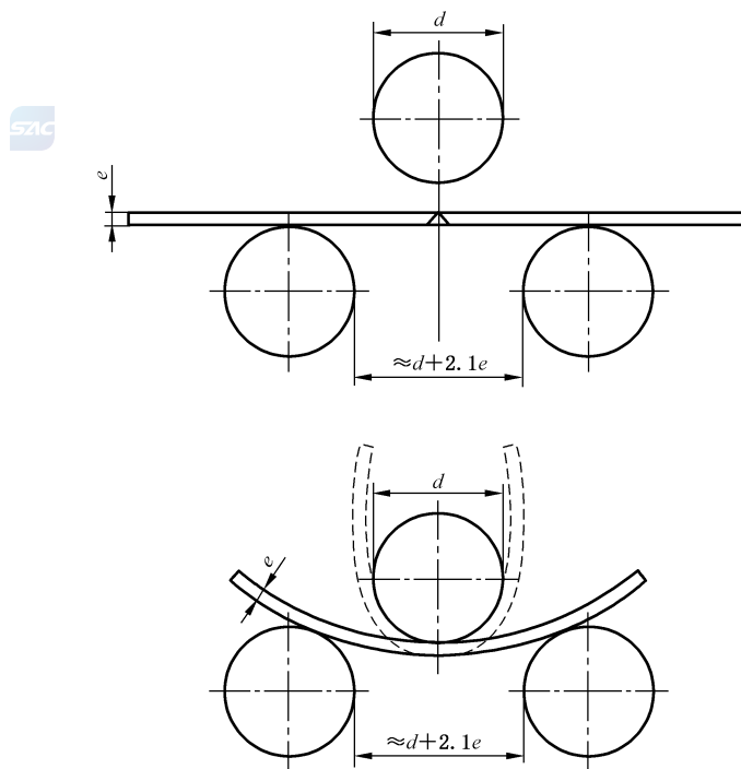
图 7 对接接头弯曲试验
